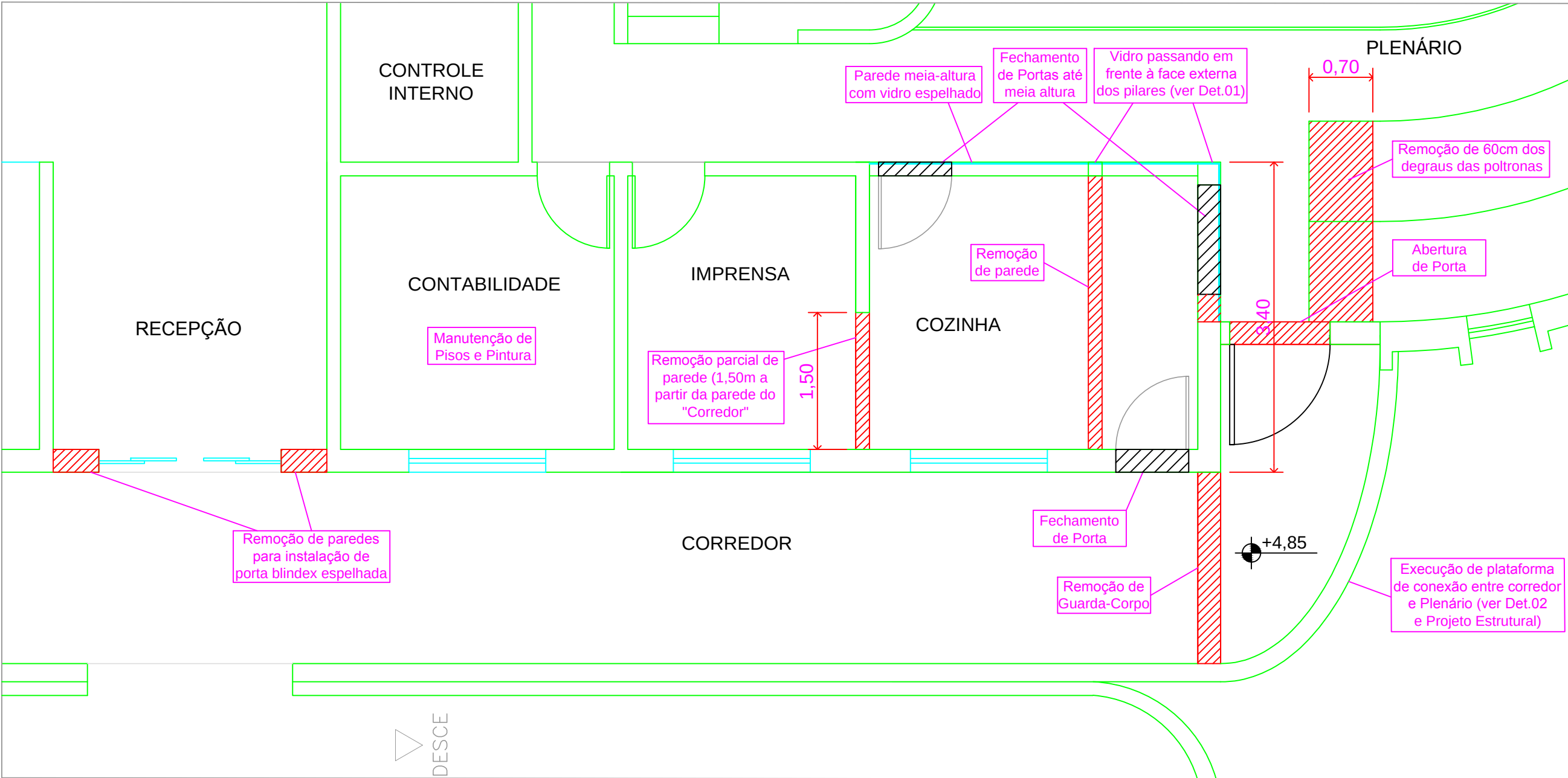
PAVIMENTO SUPERIOR - CÂMARA MUNICIPAL DE IBIÁ-MG PLANTA DE EXECUÇÃO E DEMOLIÇÃO - ÁREA SUDESTE Esc.: 1: 50
