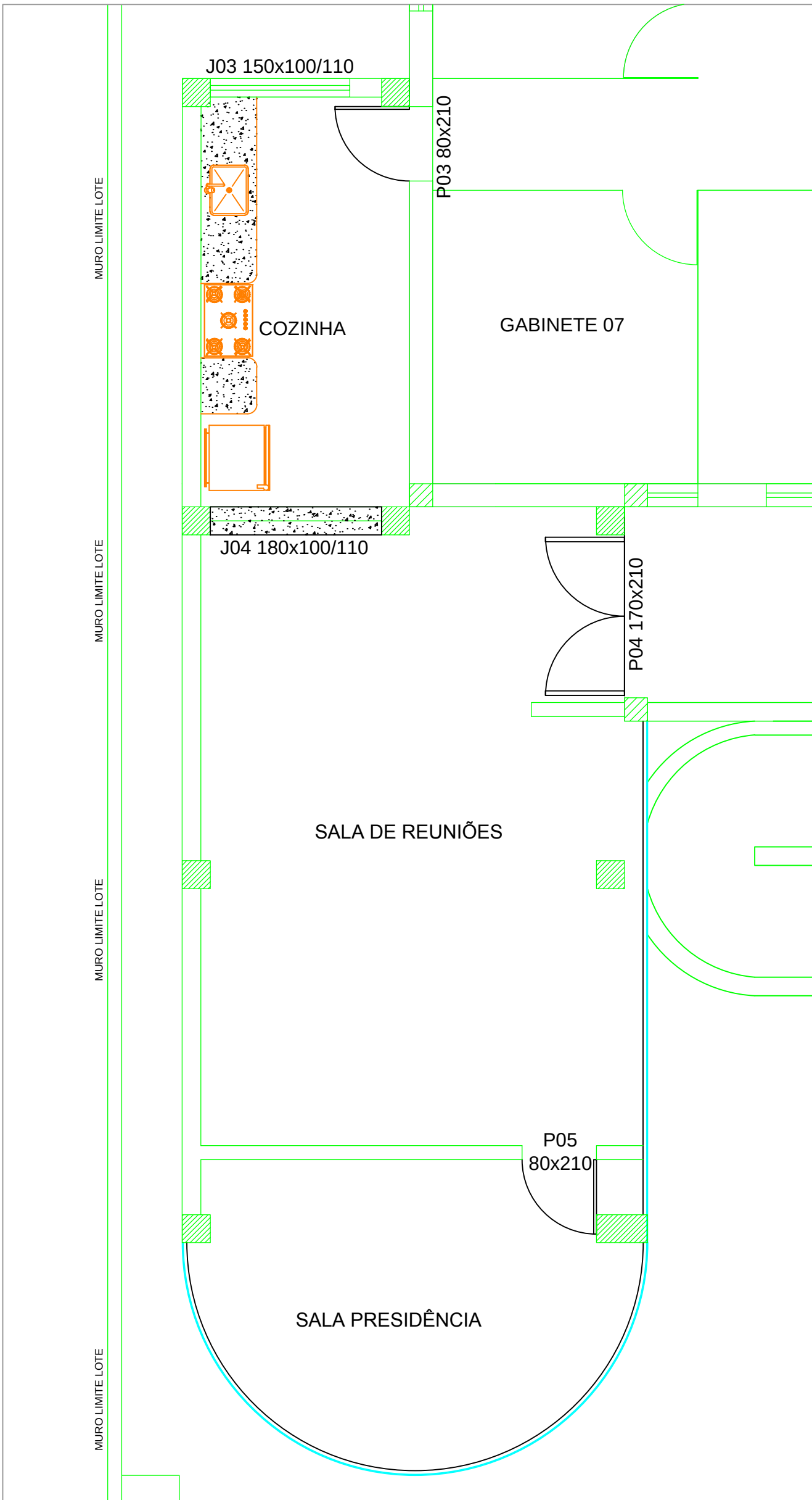
PAVIMENTO SUPERIOR - CÂMARA MUNICIPAL DE IBIÁ-MG PLANTA DO PROJETO FINALIZADO - ÁREA SUDOESTE Esc.: 1: 50
