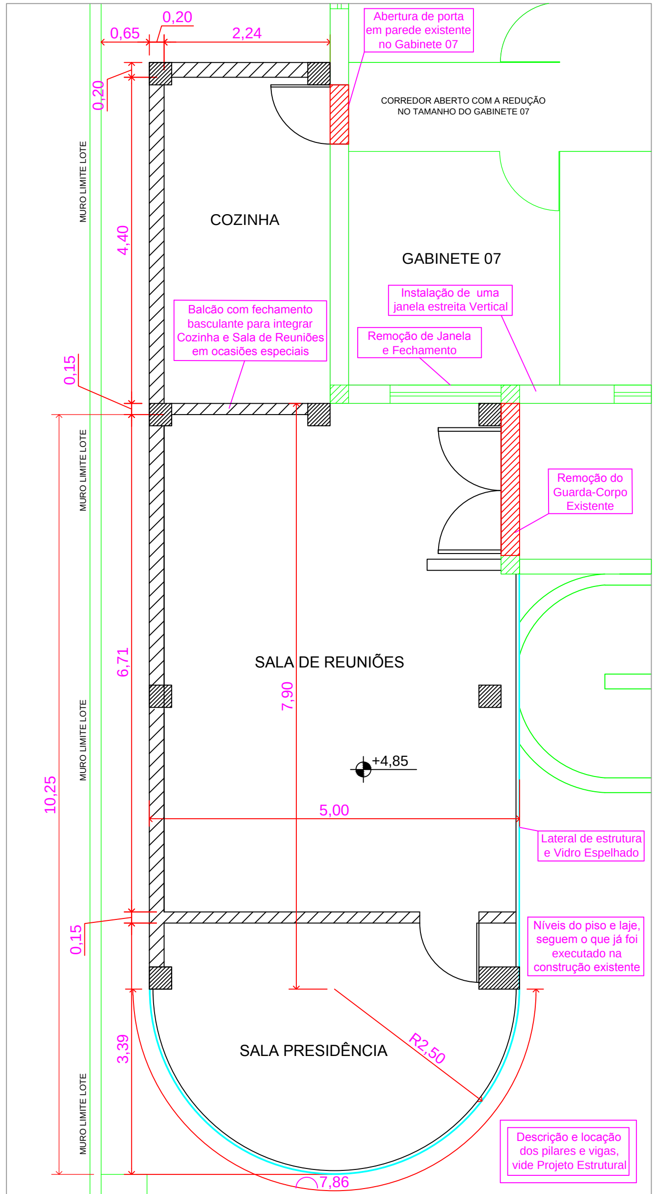
PAVIMENTO SUPERIOR - CÂMARA MUNICIPAL DE IBIÁ-MG PLANTA DE EXECUÇÃO E DEMOLIÇÃO - ÁREA SUDOESTE Esc.: 1: 50
