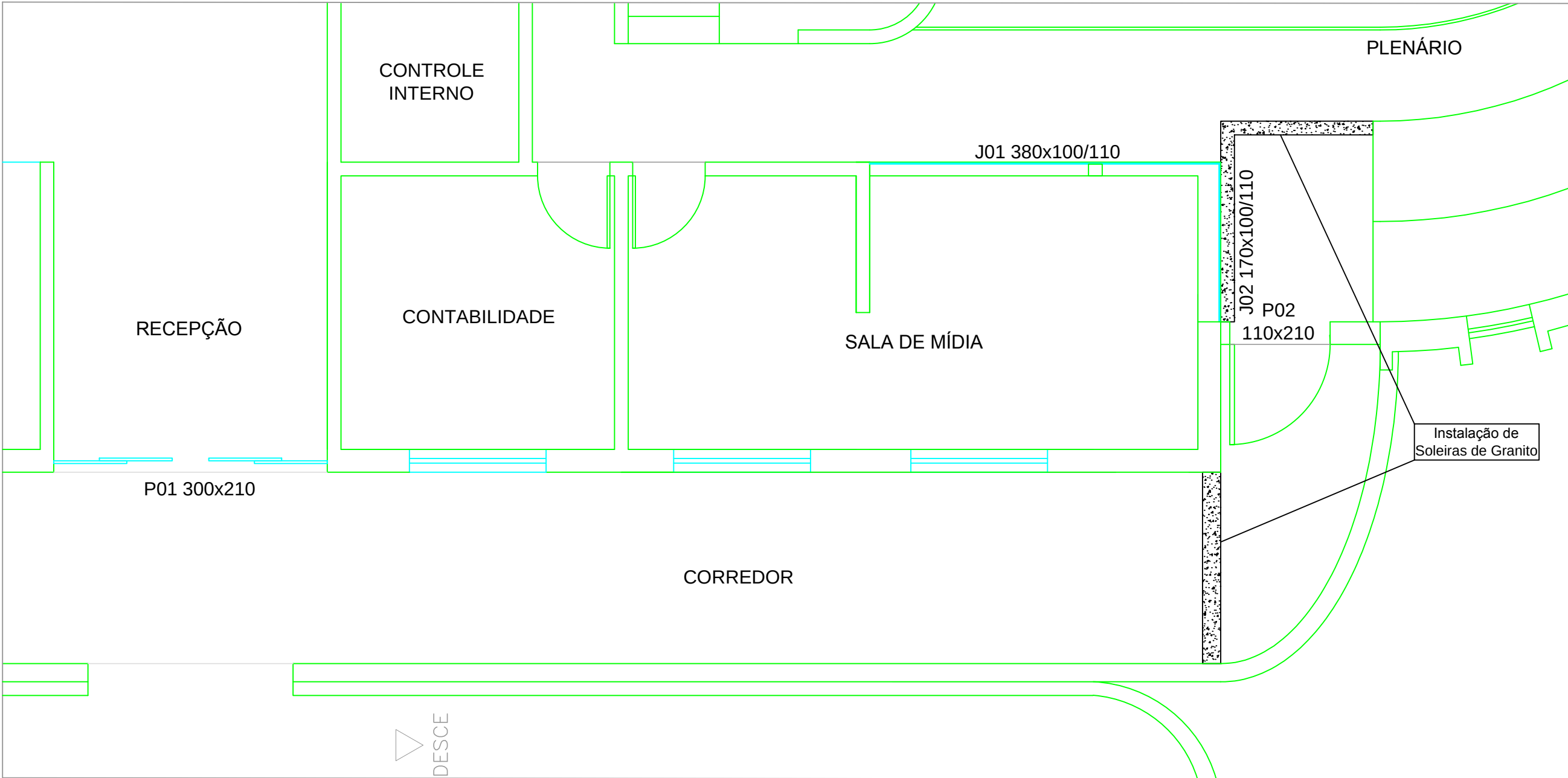
PAVIMENTO SUPERIOR - CÂMARA MUNICIPAL DE IBIÁ-MG PLANTA DO PROJETO FINALIZADO - ÁREA SUDESTE Esc.: 1: 50
